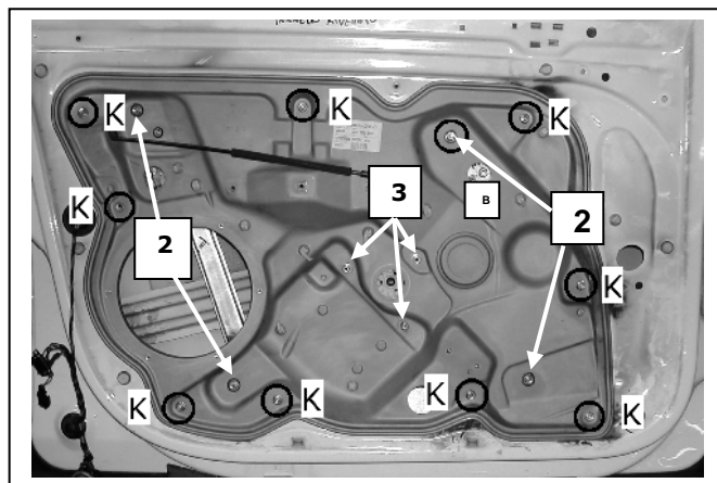
Porta lato destro, Portière avant droite, Right front door, Puerta lado derecho, Vorne rechte Tür, Porta frente dirieta, Sag on kapi, πόρτα εμπρόσθια δεξιά
