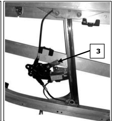
Porta lato sinistro, Portière avant gauche, Left front door, Puerta lado izquierdo, Vorne links Tür, Porta frente esquerda, Sol on kapi, πόρτα εμπρόςα αριστερή
