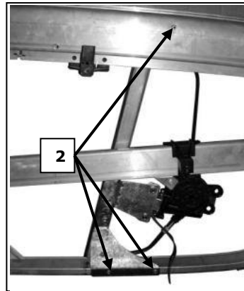
Porta lato sinistro, Portière avant gauche, Left front door, Puerta lado izquierdo, Vorne links Tür, Porta frente esquerda, Sol on kapi, πόρτα εμπρόςα αριστερή
